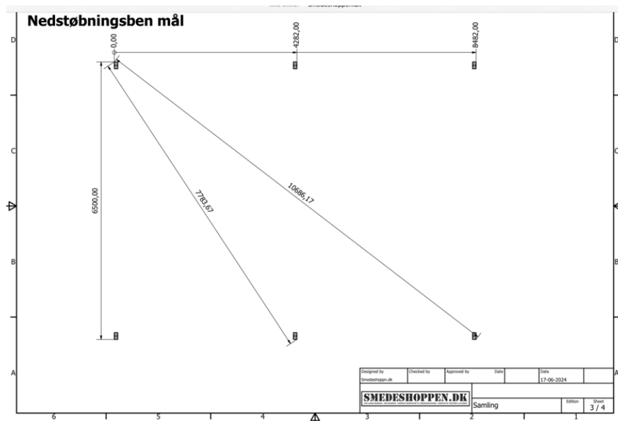
Figur 4. Nedstøbningsben mål.
